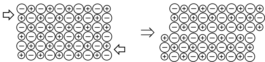
FIGURE 6.13 – Glissement des plans dans un cristal ionique
