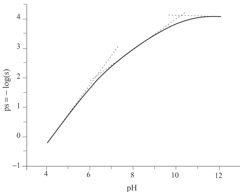
FIGURE 8.2 – Évolution de ps = f(pH)
