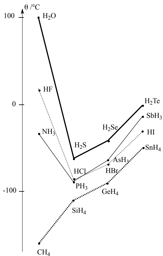
FIGURE 5.4 – Évolution des températures d'ébullition des corps purs
