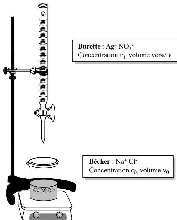
FIGURE 8.5 – Dispositif expérimental
