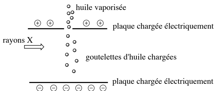
FIGURE 2.3 – Expérience de MILLIKAN
