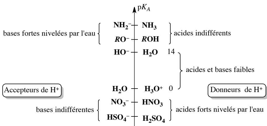
FIGURE 7.1 – Échelle d'acidité
